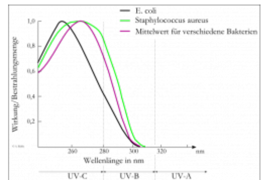
Abb. 2: Wirkungskurven für die Bakterientötung bei verschiedenen Wellenlängen, aus verschiedenen Quellen, nach Schulze, 1947
